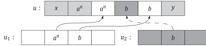
Fig. 1. u \in u_1 \sqcup u_2 .
