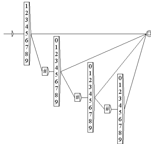
Figure 20 : Graphe Dnum9999C
