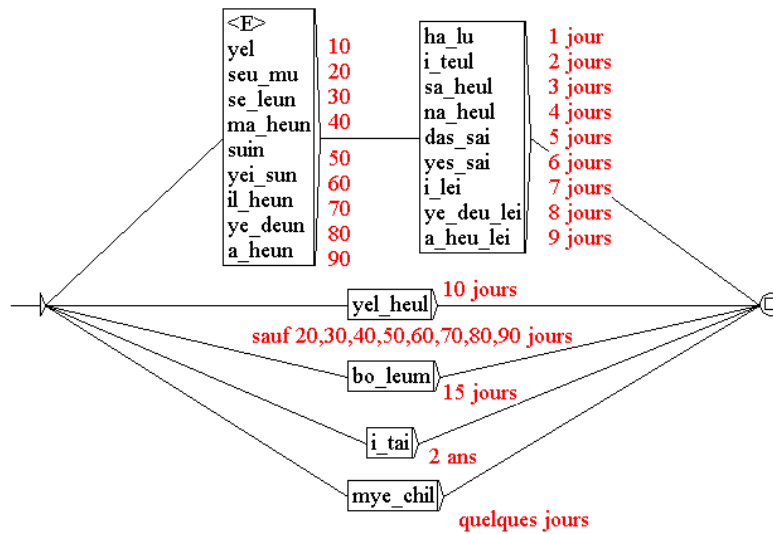
Figure 30 : Graphe NtpsSpéc
