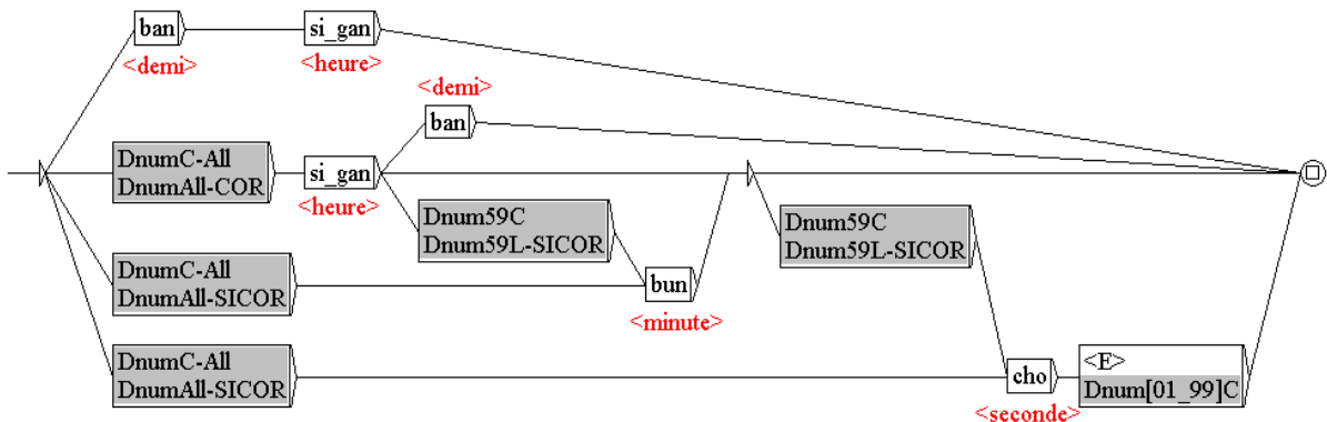
Figure 27 : Graphe HeureDurée
