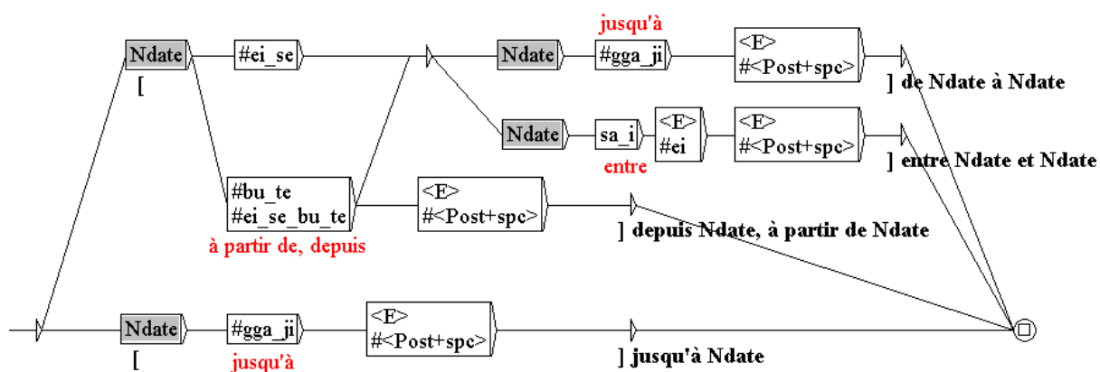
Figure 47 : Graphe bute-ggaji
