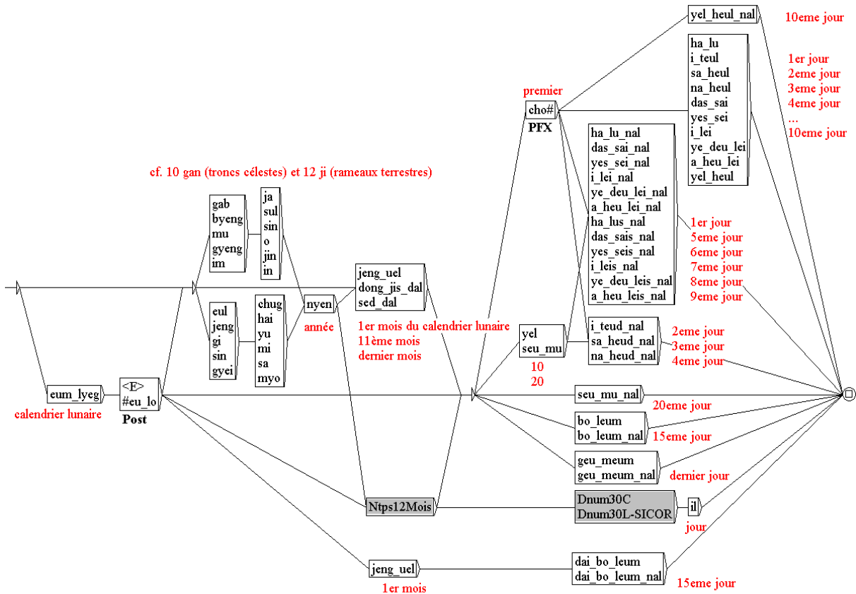
Figure 67 : Graphe AnMoisJourDate(lunaire)
